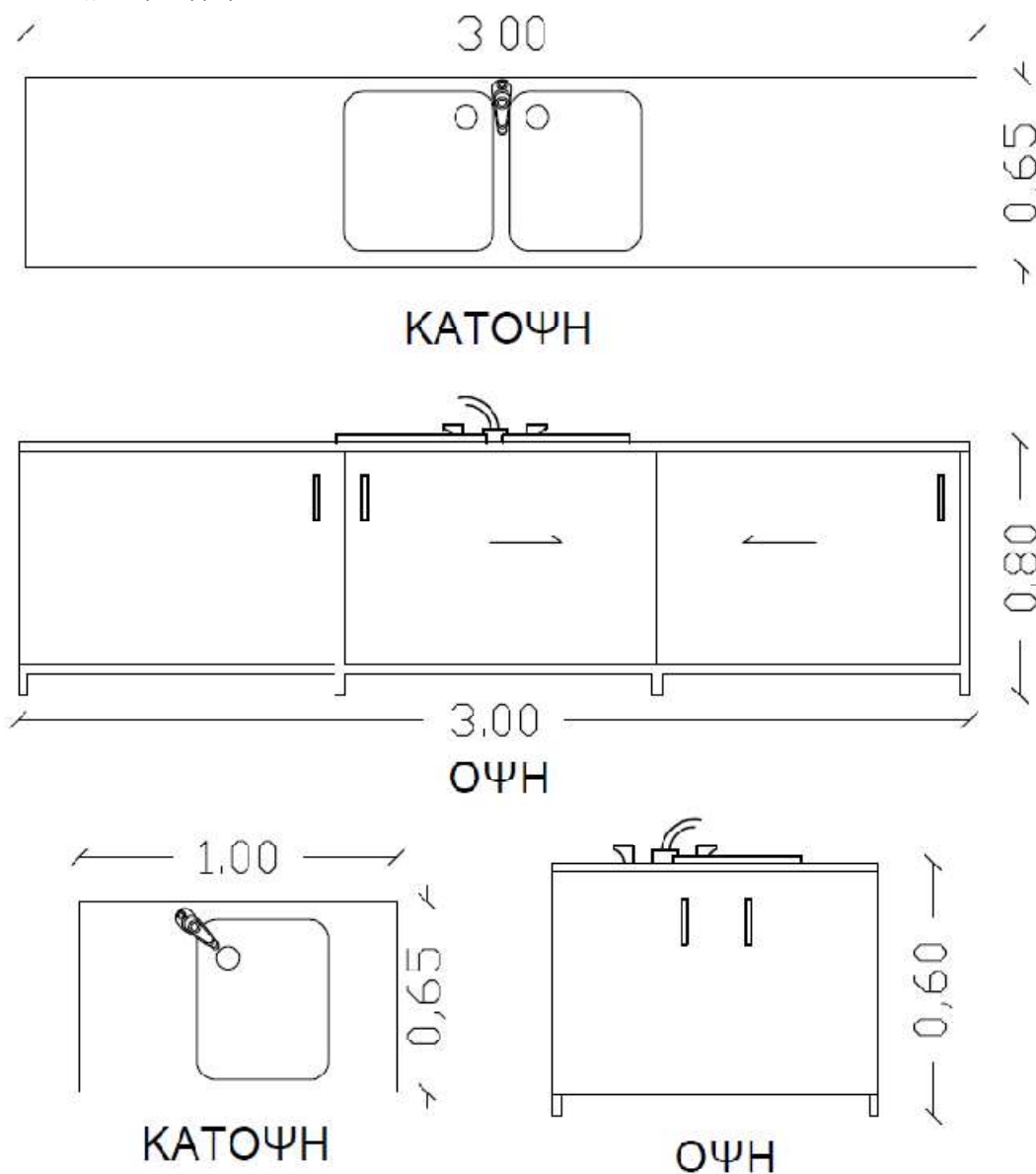
ΠΑΡΑΡΤΗΜΑ Α': Σχέδιο για ερμάρια
