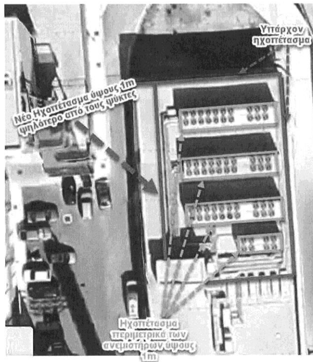
Ενδεικτική θέση ηχομονωτικών επεμβάσεων στις Η/Μ εγκαταστάσεις του δώματος
